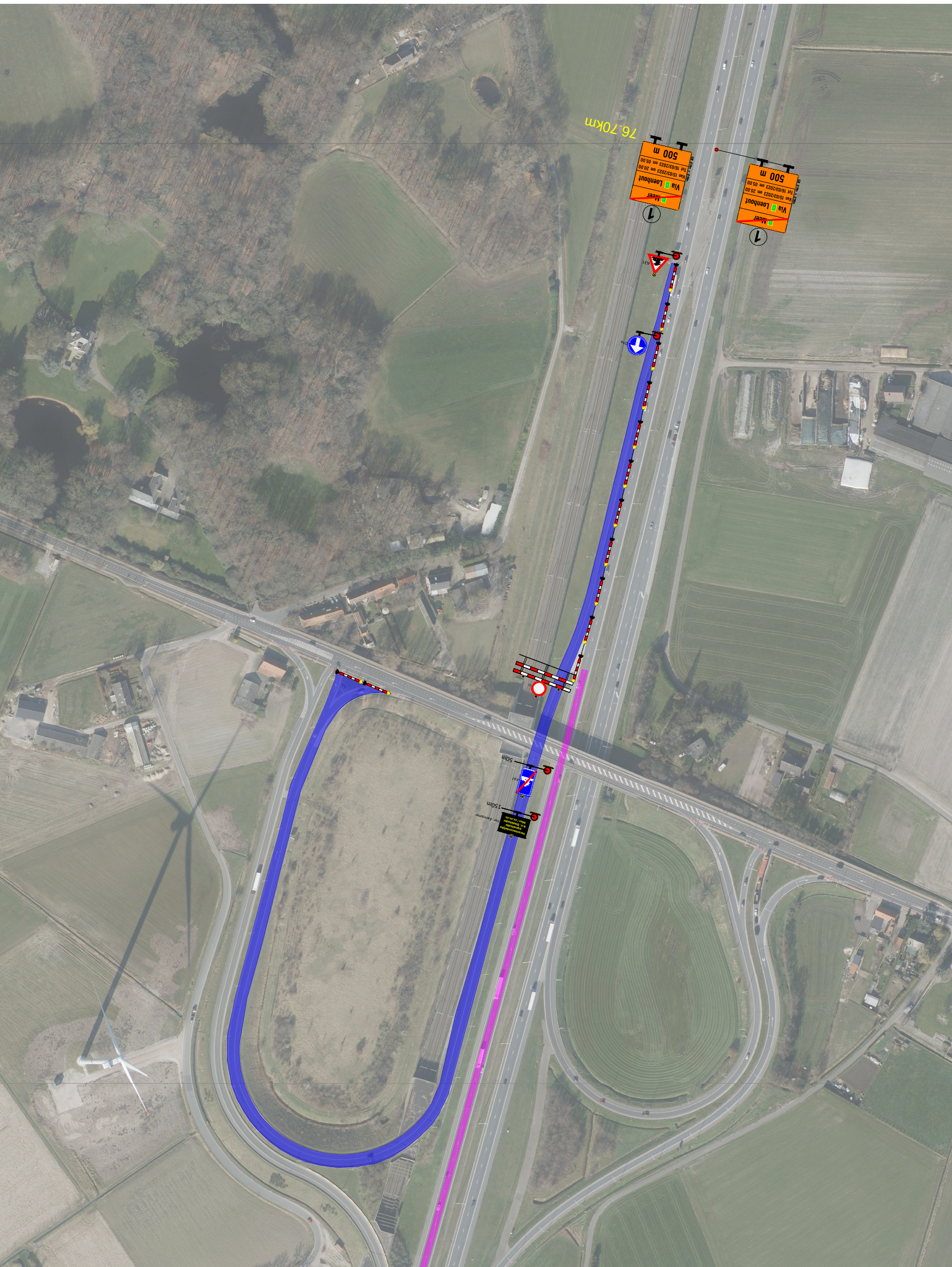
Omleidingsplan afsluiting afrit 1 Meer
